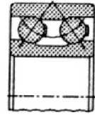
Двухрядный с цельными кольцами
