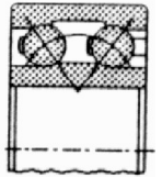
Двухрядный с цельными кольцами
