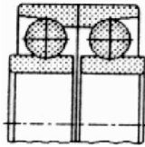
Сдвоенные с двумя бортами на внутреннем кольце, углом контакта 12°, наружные кольца обращены друг к другу широкими торцами
