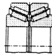
Двухрядный с двумя внутренними кольцами и цельным наружным кольцом
