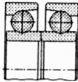
Сдвоенные с двумя бортами на внутреннем кольце, углом контакта 12°, наружные кольца обращены друг к другу узкими торцами
